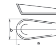
Lodička spalovací s ouškem Combustion boat with eyelet Verbrennungsschiffchen mit Henkel Barquilla para combustión con orejuela Лодочка для сжигания с ушком
